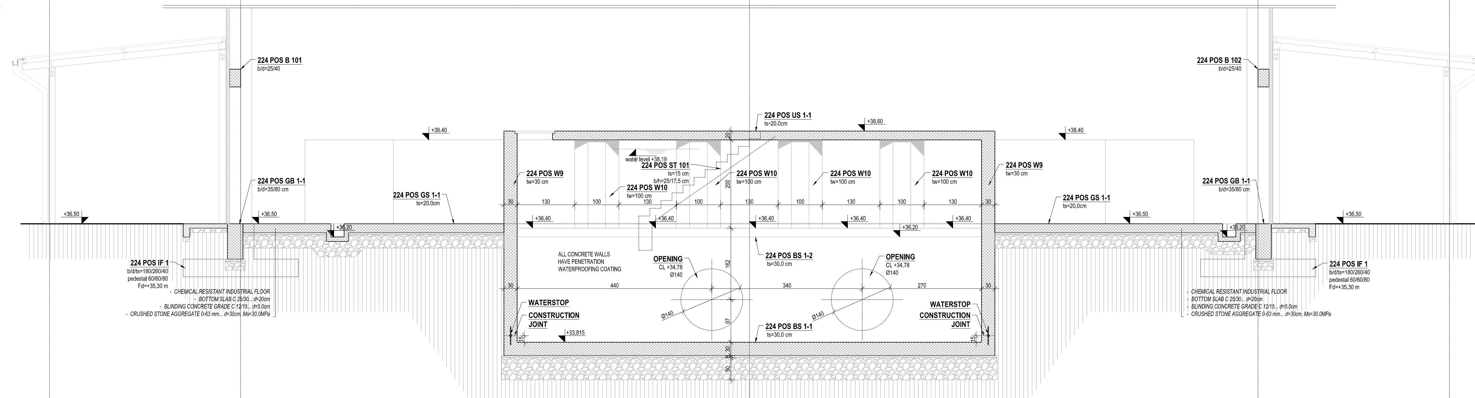
SECTION A-A
